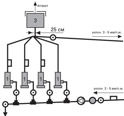
Рис. 2 Параллельное подключение. Эл. механический вариант автоматики.
